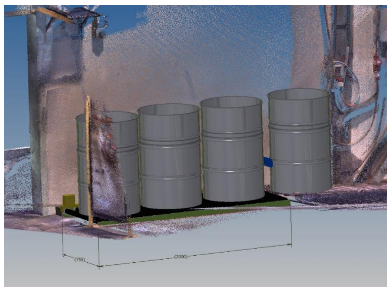
ESEMPIO DI QUOTATURA DELL'ASSIEME REALIZZATO
